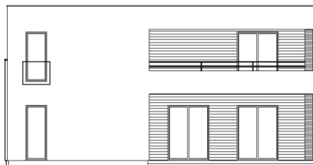
ELEWACJA WSCHODNIA
