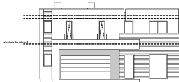
ELEWACJA ZACHODNIA
